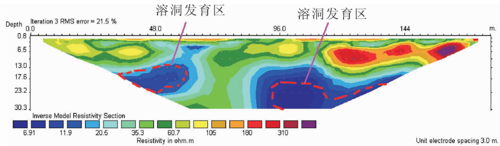
图 3 杭州丝绸博物馆电阻率断面图 Fig.3 Resistivity profile of Hangzhou Silk Museum
