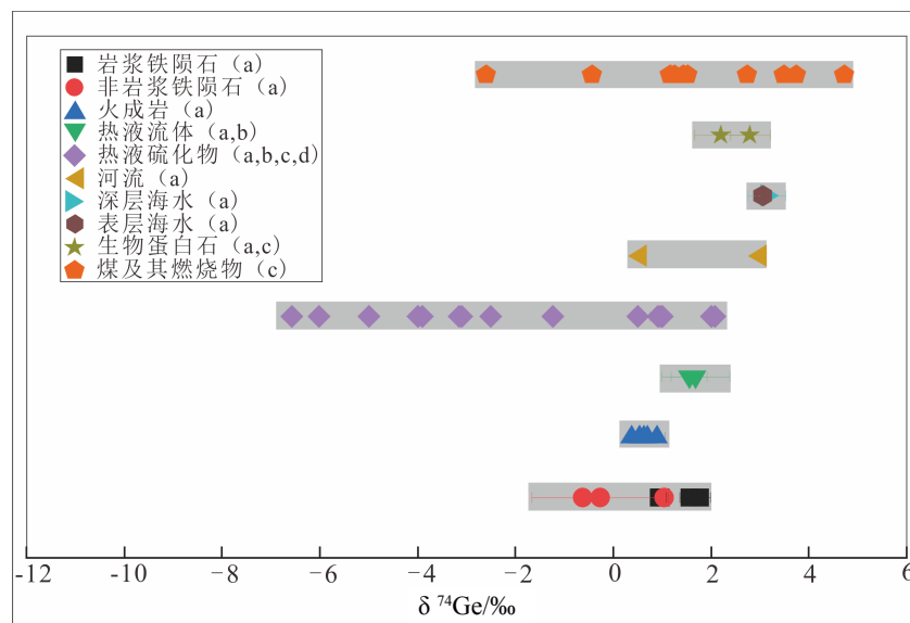
①a据Rouxel等(2017);②b据Luais等(2014);③c据孟郁苗(2014);④d据Liu等(2020)
