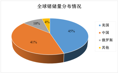
图4 全球锗储量分布情况图 (数据来源:中商产业研究院整理)
