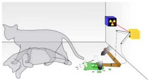
图1 薛定谔的猫
