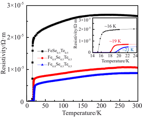
图8 \text{Fe}_x\text{Se}_{0.5}\text{Te}_{0.5} 电阻率与温度的关系曲线
