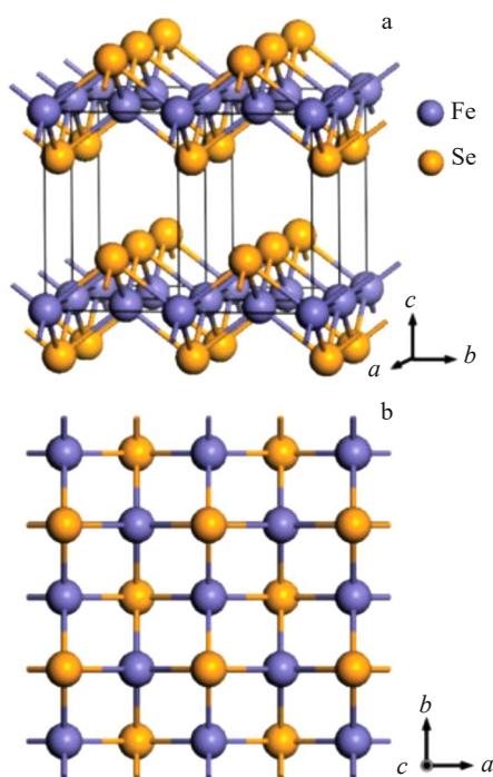
图1 \beta -FeSe 晶体结构示意图和俯视图
