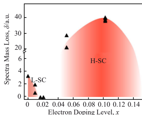
图 10 超导电性与电子掺杂水平 x 的相关性
