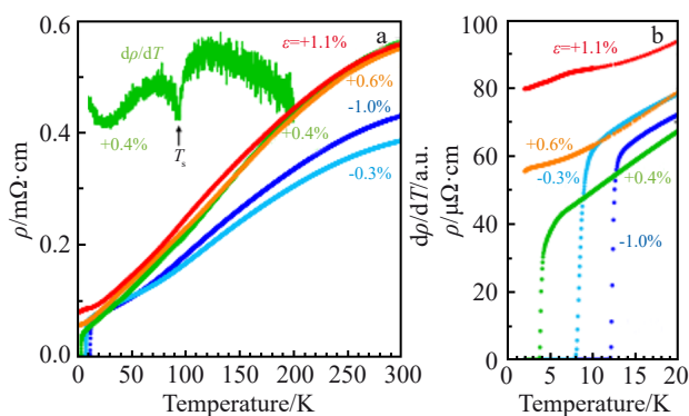
图7 不同应变下FeSe薄膜直流电阻率 \rho 的温度依赖性和超导转变温度附近FeSe薄膜电阻率的温度依赖性
