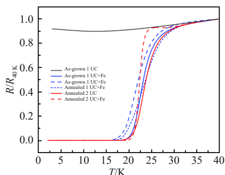
图11 不同样品的归一化电阻随温度变化关系
