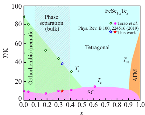
图3 块状 \text{FeSe}_{1-x}\text{Te}_x 超导体的 T_c - x 之间的相图
