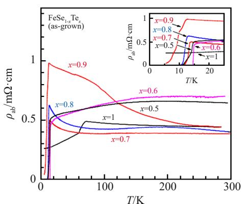
图2 \text{FeSe}_{1-x}\text{Te}_x 单晶 ( 0.5 \leq x \leq 1 ) 面内电阻率的温度依赖性
