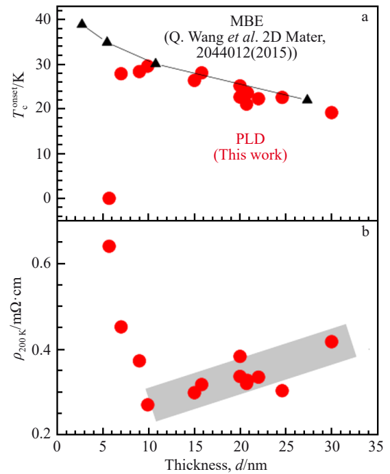
图5 FeSe/STO薄膜的起始 T_c 与厚度的关系和薄膜在200 K下电阻率的厚度依赖性
