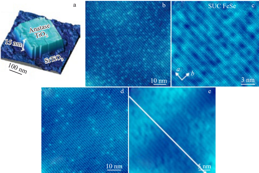
图9 FeSe/ \text{TiO}_2 (001)结构示意图、退火前 \text{TiO}_2 的STM形貌、退火前1-UC FeSe膜的原子分辨STM形貌、750 °C退火后 \text{TiO}_2 的STM形貌和退火后1-UC FeSe膜的原子分辨STM形貌
