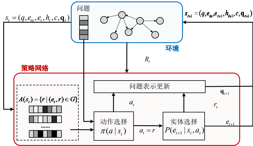
图 3.1 约束路径推理模型框架
