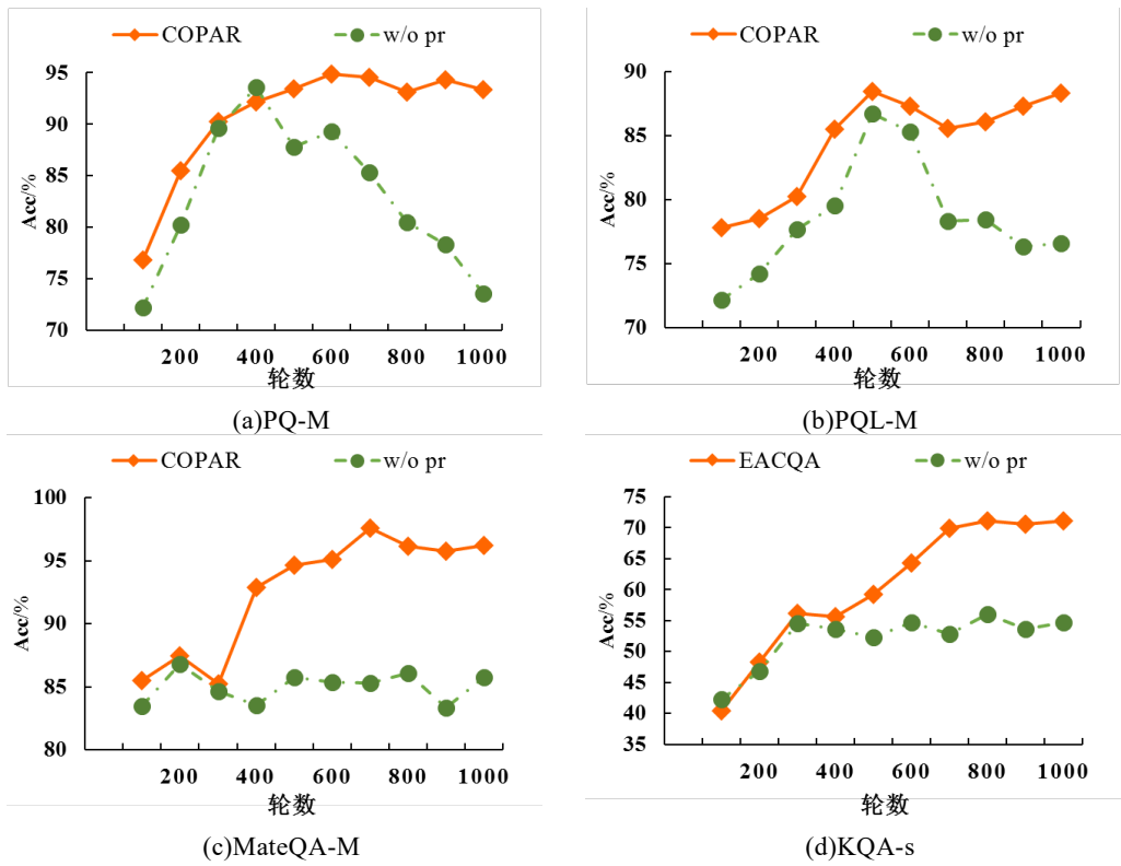
图 4.2. 基于潜力的塑形奖励函数对整体模型的有效性验证
