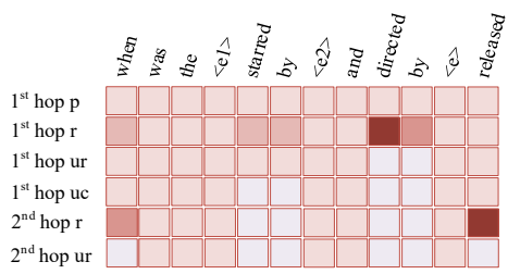
图 4.1. 问题更新过程示例
