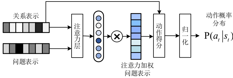
图 3.2 动作选择策略网络
