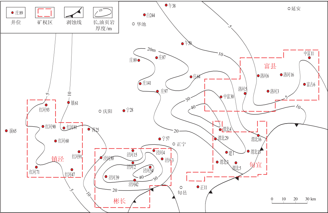
图5 鄂尔多斯盆地南部延长组长7油页岩厚度平面分布
