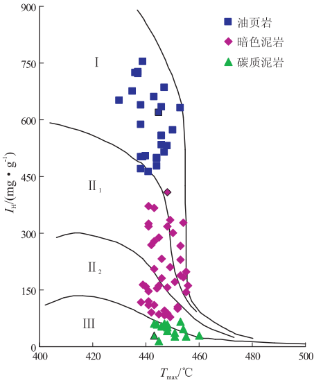
图 2 鄂尔多斯盆地南部延长组不同岩性烃源岩有机质类型
