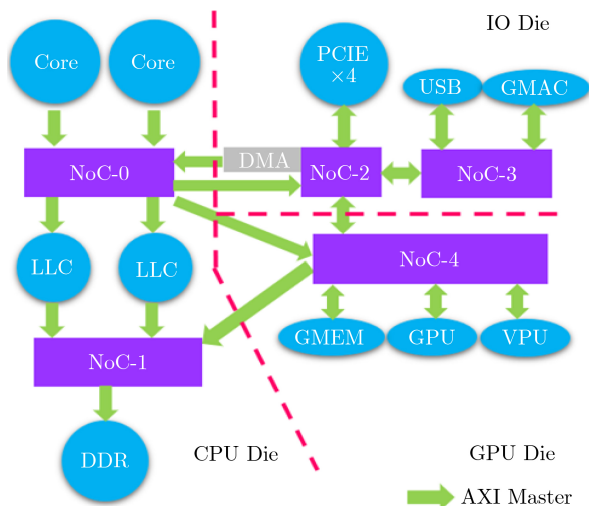
图1 MSoc芯片架构图
