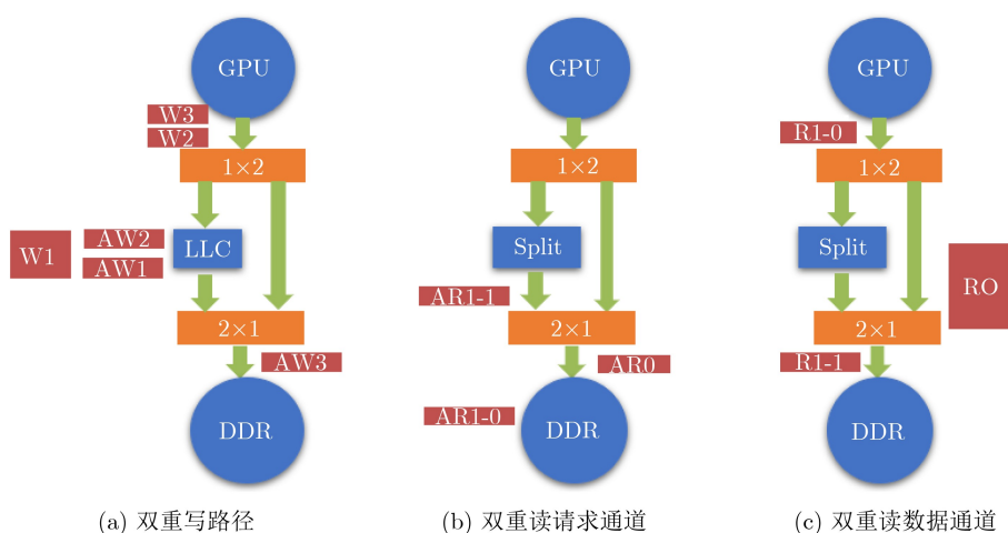
图2 双重路径死锁图示
