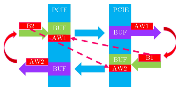
图4 桥接死锁图示
