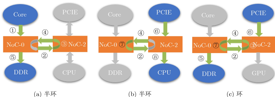
图3 环形通路死锁图示
