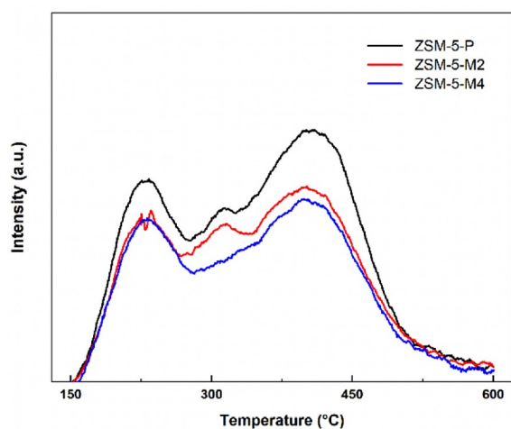
图3 不同沉积量及原始的ZSM-5分子筛的氨气程序升温脱附曲线(网络版彩图)
