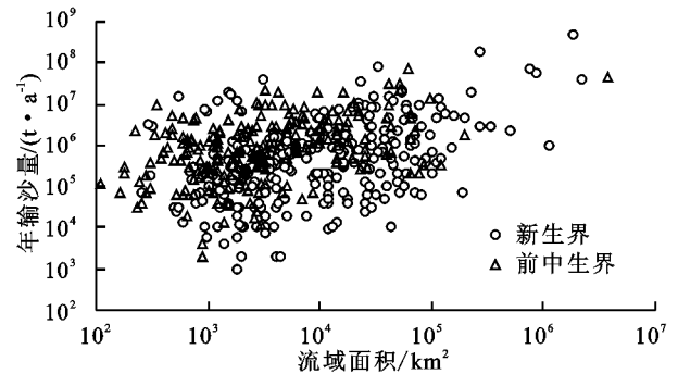
图 2 流域面积—输沙量关系
