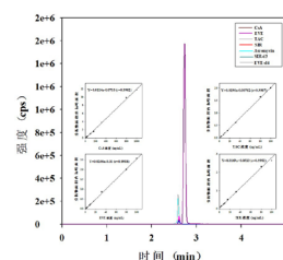
4 种免疫抑制剂色谱图及线性
