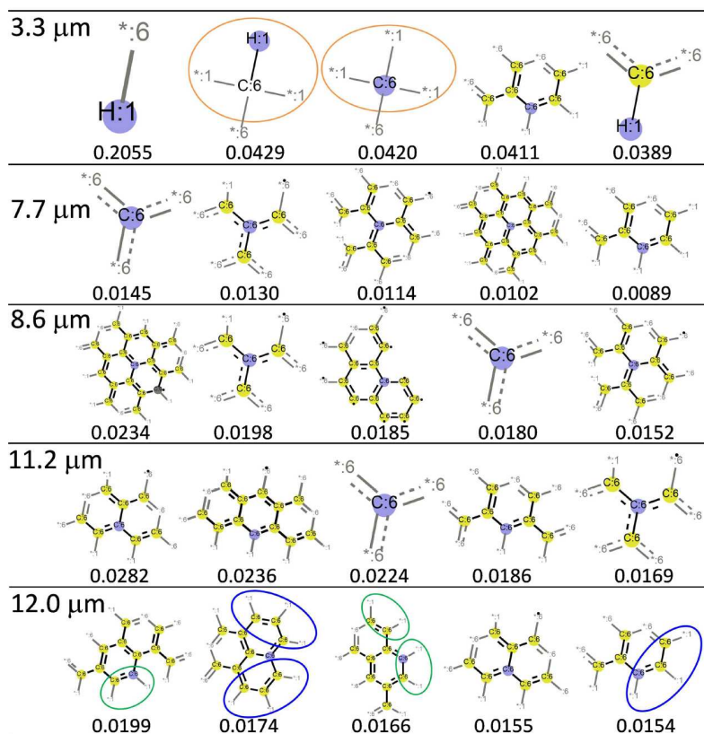
图 7 (网络版彩色)不同红外波段的主要分子片段及其重要性排序 [34] . 展示了3.3、7.7、8.6、11.2和12.0 μm红外波段的5个最重要分子片段, 按其特征重要性值从高到低排序. 这些分子片段是通过机器学习分析确定的, 反映了它们在各波段的贡献程度
