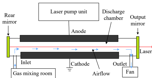
图 1 激光器系统截面示意图
