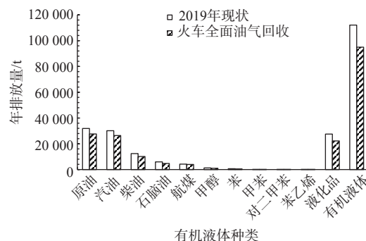
图 3 2022 年完成火车油气回收减排量的预测
