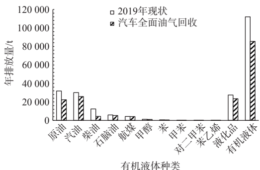
图 4 2022 年完成汽车油气回收减排量
