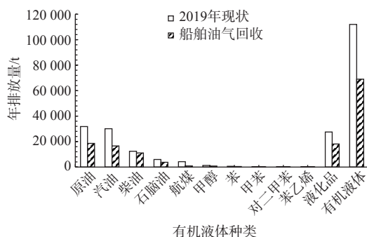
图 2 2022 年全年完成船舶油气回收减排量预测
