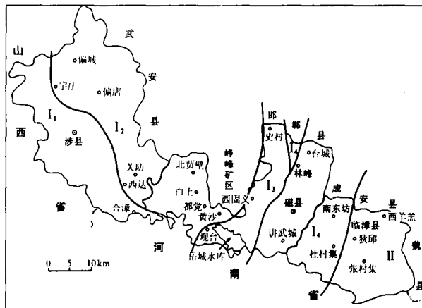
图 1 河北省南部地区食管癌分布图
