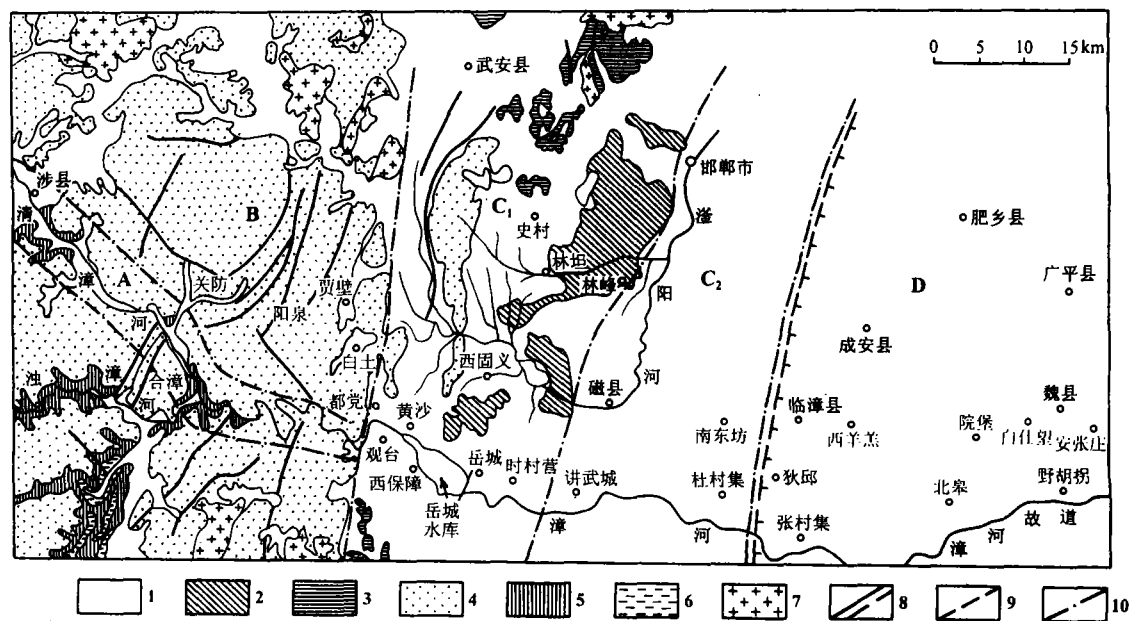
图2 研究区地质及地质生态环境分区图
