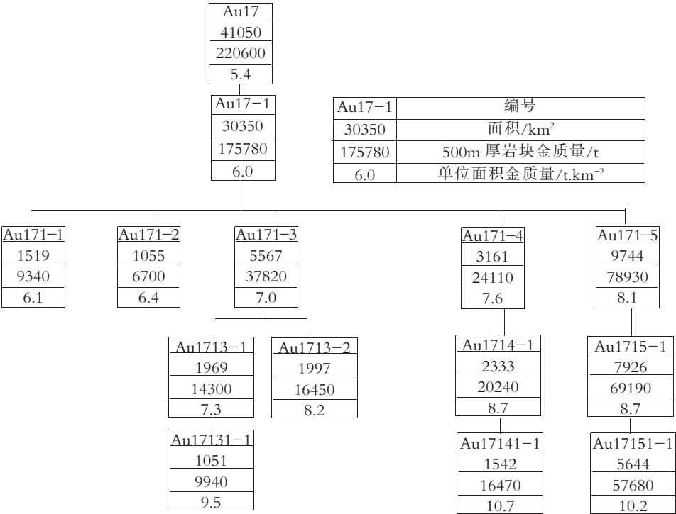
图 3 西秦岭东部 Au 地球化学块体内部结构谱系图
