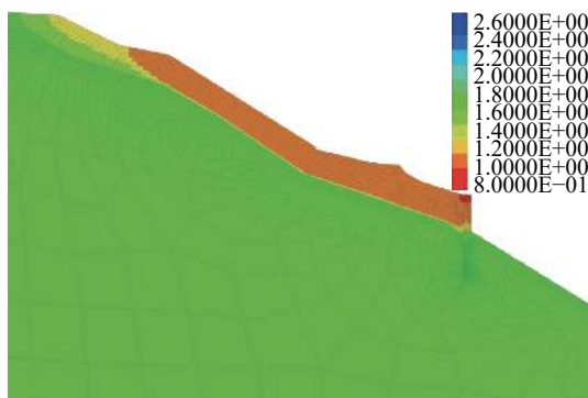
图 15 失去支挡后罕遇地震工况下滑坡稳定性分区云图
