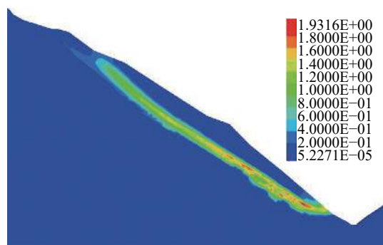
图 11 沟道现状条件下滑坡前缘最大剪应变增量云图
