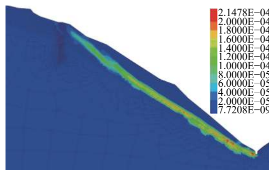
图 7 坡脚下切后斜坡最大剪应变增量云图
