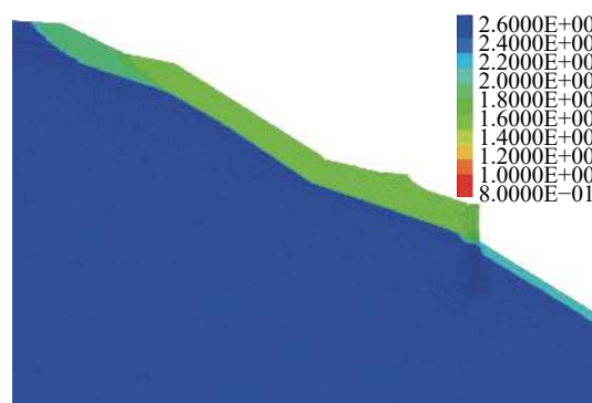
图 12 失去支挡后天然工况下滑坡稳定性分区云图
