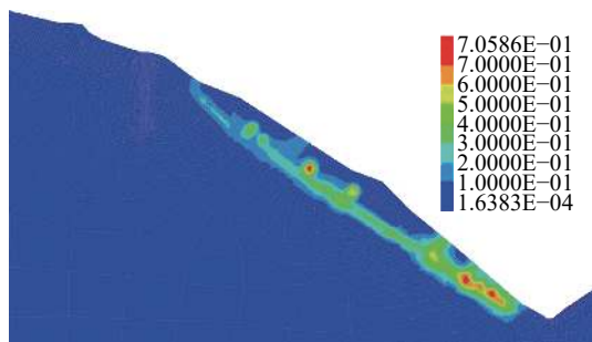
图 6 多遇地震条件下斜坡最大剪应变增量云图
