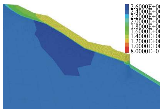
图 14 失去支挡后基本地震工况下滑坡稳定性分区云图
