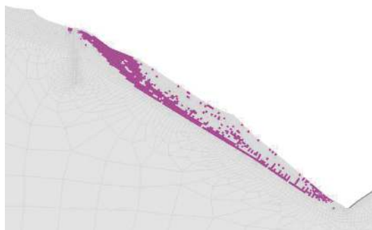
图 5 多遇地震条件下斜坡塑性区发育分布图
