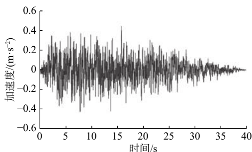
图 4 多遇地震条件下人工合成地震波时程曲线
