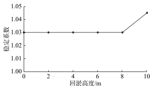
图 10 不同回淤高度滑坡前缘稳定系数变化情况
