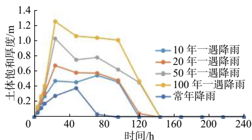
图 8 距离 240 m 处强降雨历时全过程饱和土体厚度变化情况 (2-2' 剖面)
