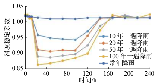
图 9 滑坡体在强降雨入渗条件下稳定系数变化情况
