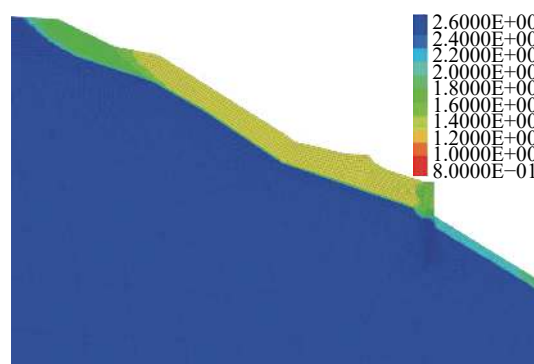
图 13 失去支挡后多遇地震工况下滑坡稳定性分区云图
