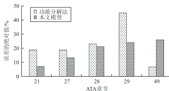
图4 不同模型计算误差的绝对值
