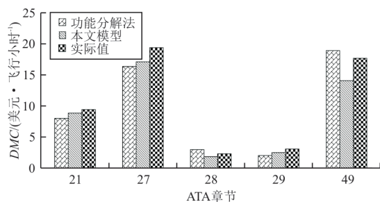
图3 模型计算值与实际值对比
