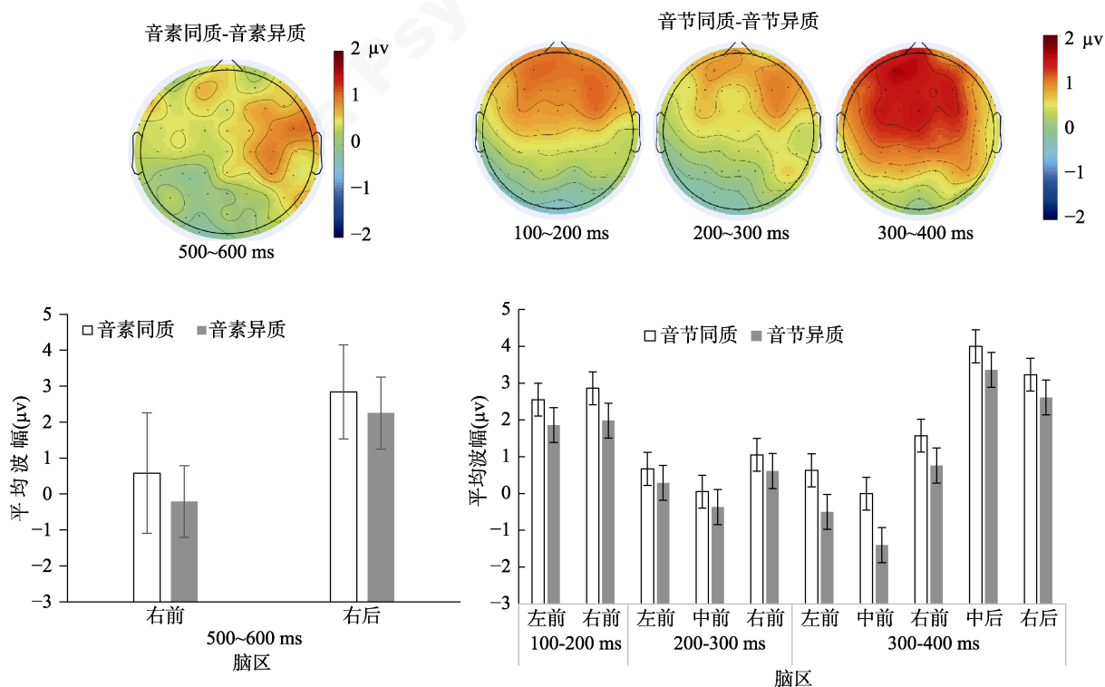
图 3 在不同时间窗口下的音节和音素效应的平均波幅与各个时间窗口下的地形图(图中误差棒均为 95% CI)
