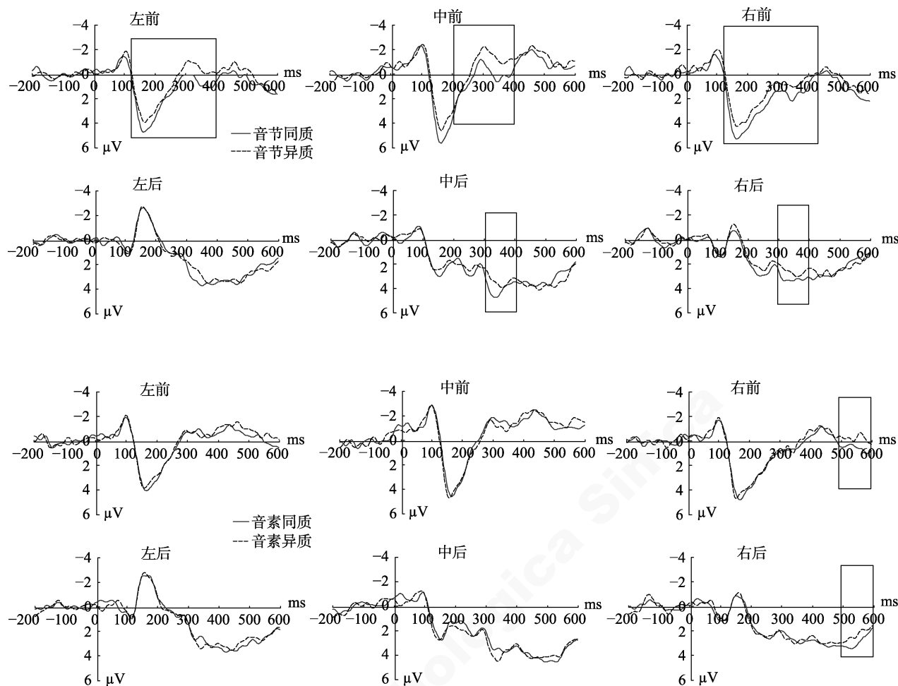
图 2 6 个兴趣区内音节和音素效应的平均波形图(方形框表示两类条件对比有显著差异)
