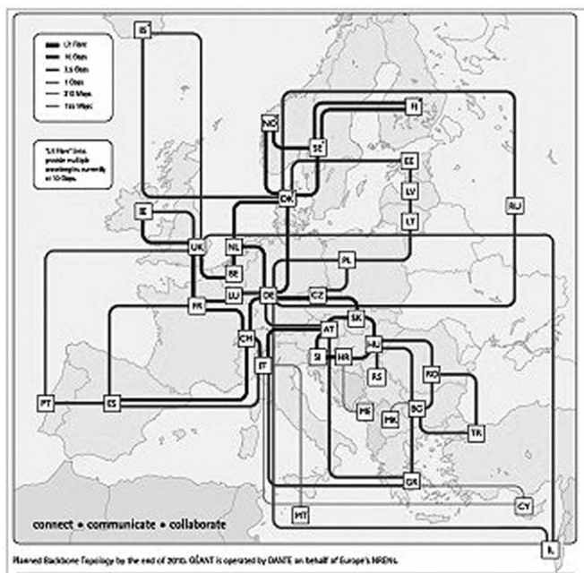
图2 欧洲 GÉANT2 主干网拓扑
