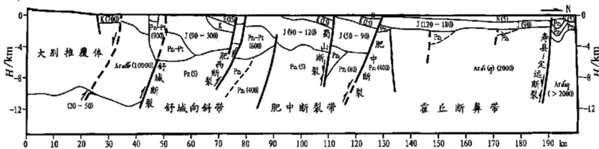
图2 合肥盆地南北向电性-地质解释剖面 (括号内为电阻率数据, 单位 \Omega\cdot\text{m} )
