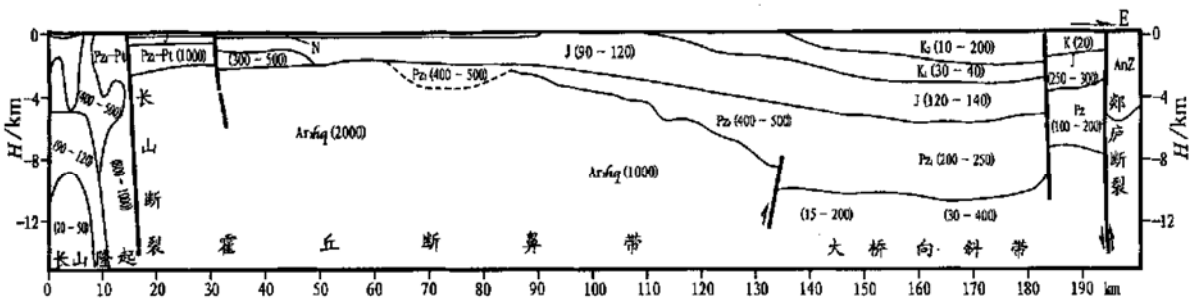
图3 合肥盆地北部东西向电性-地质解释剖面 (括号内为电阻率数据, 单位 \Omega\cdot\text{m} )
