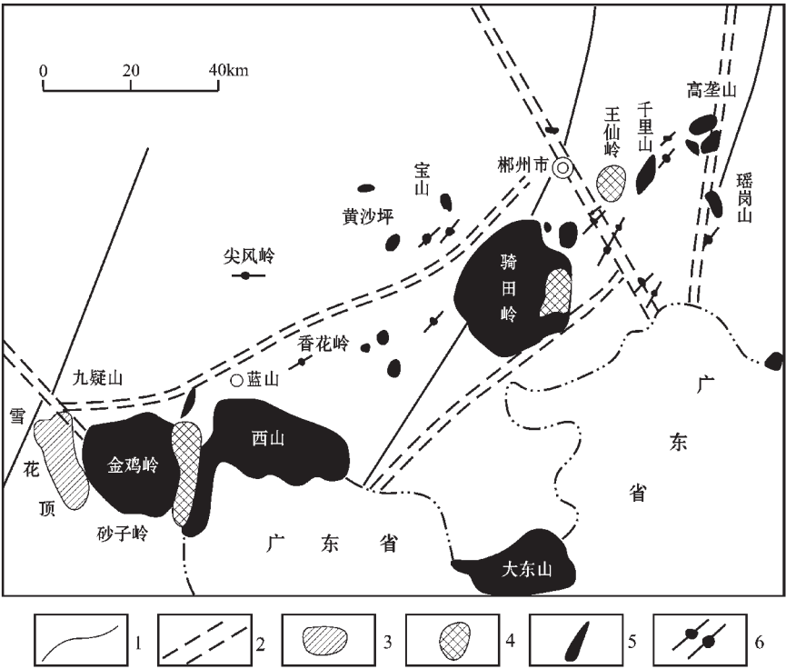
图6 郴州—蓝山构造岩浆岩带略图
