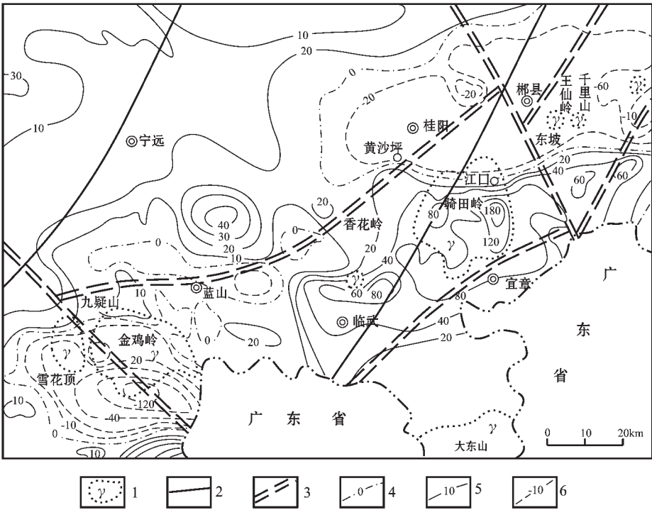
图3 郴州—蓝山构造岩浆带航磁ΔT异常图
