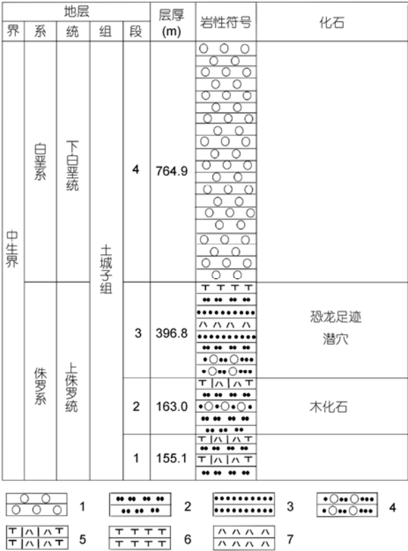
图 2 延庆县土城子组地层柱状图
