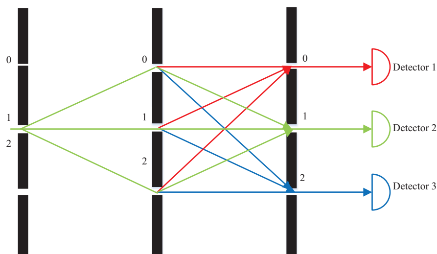
图 2 (网络版彩图) 三狭缝的对偶量子计算机演示图. 从标记为 1 的第 2 个狭缝输入, 和由中间屏幕的 3 个狭缝分为 3 个子波. 中间屏幕后, 在不同的狭缝对子波进行不同的操作. 对偶量子计算的输出从右边屏幕上的 3 个狭缝处获得, 不同的狭缝处的输出对应不同的量子计算结果
