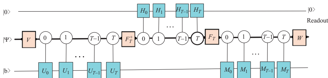
图 5 (网络版彩图)HHL 算法的对偶量子线路图. 我们只需要辅助比特处在 |0\rangle 时系统输出结果
