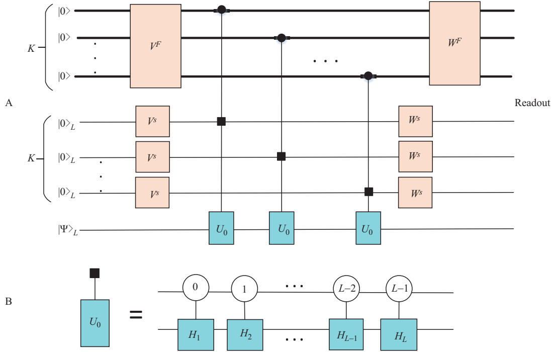
图 4 (网络版彩图)BCCKS 算法的对偶模式量子线路图. A 展示的是整个线路图. 其中 |\Psi\rangle 是工作系统初态. 线路图共包含 K 个 |0\rangle 态的辅助控制比特和 K 个 L 能级的 |0\rangle_L 辅助控制系统. B 展示的是 U_0 由 H_1, H_2, \dots, H_{L-1}, H_L 组成. 只有当处在圆圈内相应的态的时候辅助系统控制的幺正算符 U_0 才会被激发
