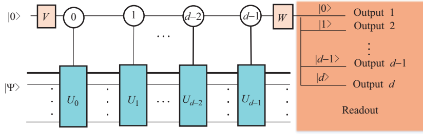
图 3 (网络版彩图) 多输出的对偶量子计算线路图. |\Psi\rangle 是工作比特初态, |0\rangle 是辅助比特初态
