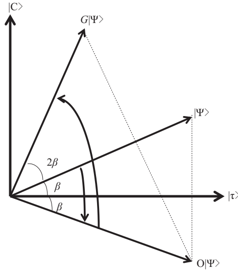
图 1 Grover 搜索算法的几何示意图, 修改自参文 [36]
