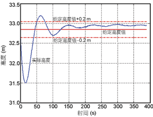
图 2 自动定高
