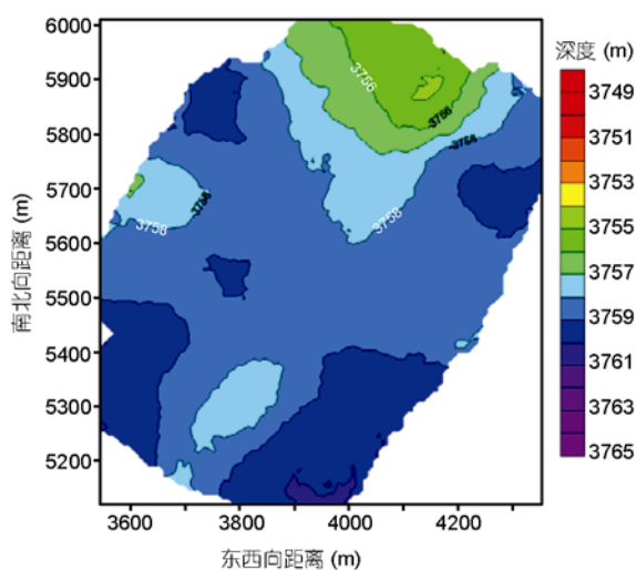
图3 海底测绘
