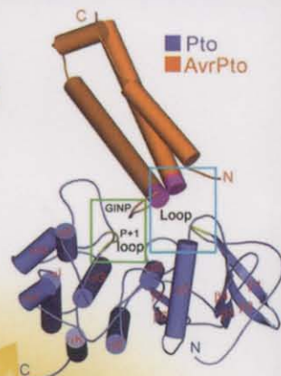
细菌效应蛋白AvrPto和 植物中对应的抗性蛋白 Pto的复合物晶体结构
