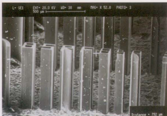
采用LIGA技术的深度X光光刻大深宽比结构
