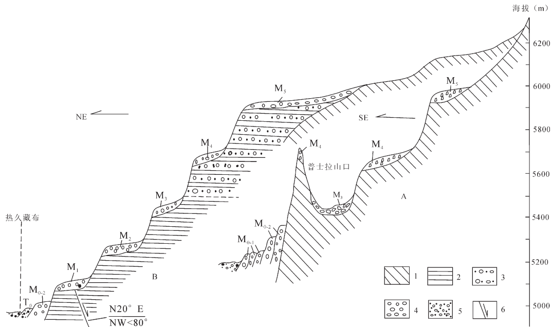
图 3 卓奥友峰北麓热久藏布谷地左侧综合地貌横剖面
