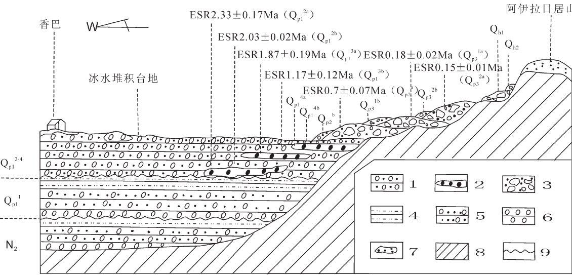
图 5 扎达盆地香巴—阿伊拉日居山第四纪冰川堆积示意剖面 [10]
