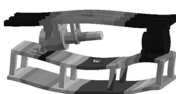
图 9 第 6 阶振型(上下振动)
