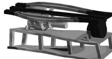
图 8 第 5 阶振型(结构扭转)
