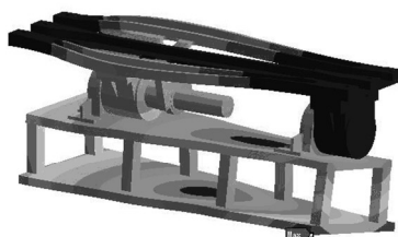
图 5 第 2 阶振型(结构扭转)
