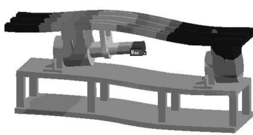
图 7 第 4 阶振型(上下振动)
