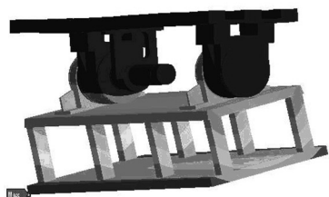
图 4 第 1 阶振型(减速器扭转振动)
