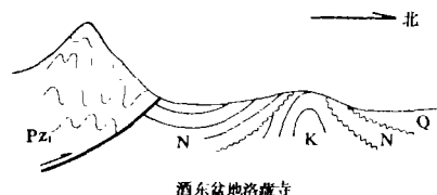
图4 酒东盆地祁连山大断裂示意图
