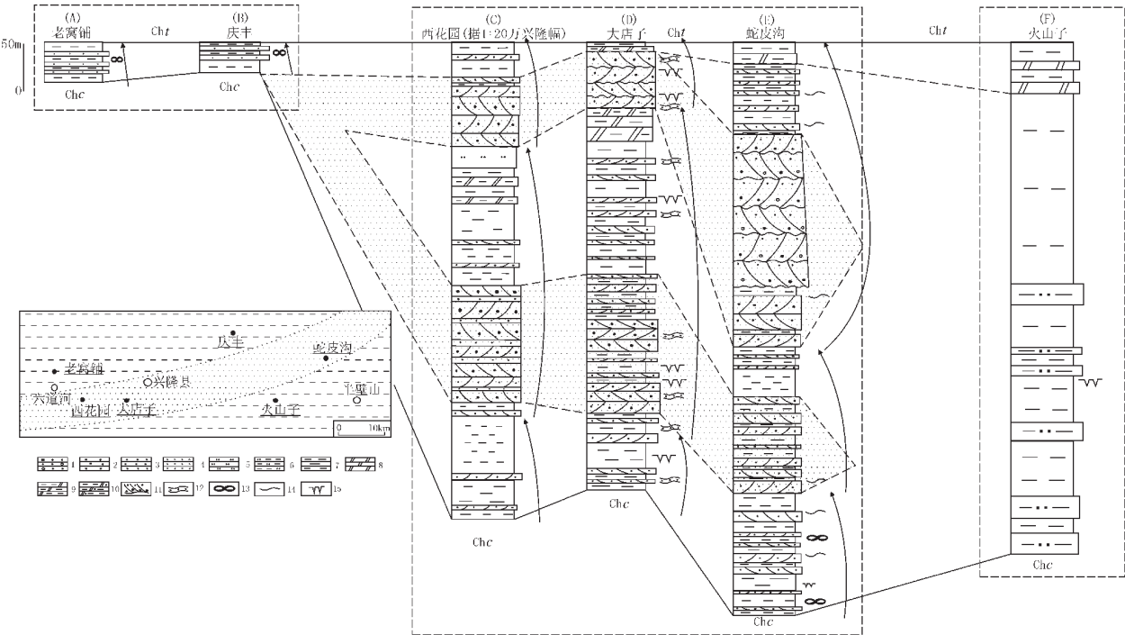
图2 兴隆地区串岭沟组地层对比
