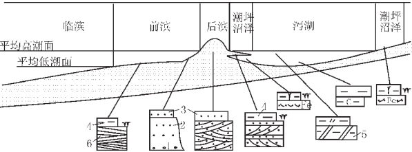
图3 串岭沟组米级旋回类型与环境变化谱系
