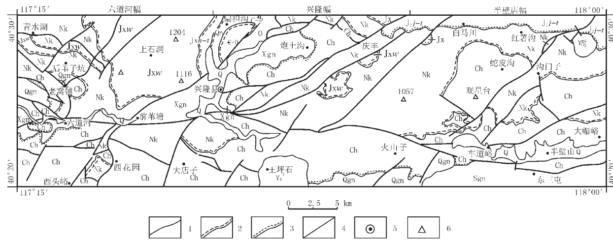
图1 研究区地质构造略图
