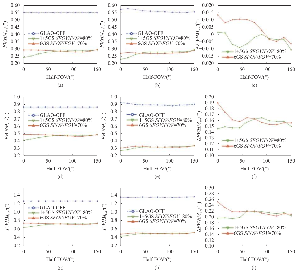
图 6 不同湍流环境下各视场环带平均校正效果图, 其中“o”虚线代表开环, “Δ”与“▽”分别代表导引星呈单环与双环“1+5”下系统闭环校正效果。
