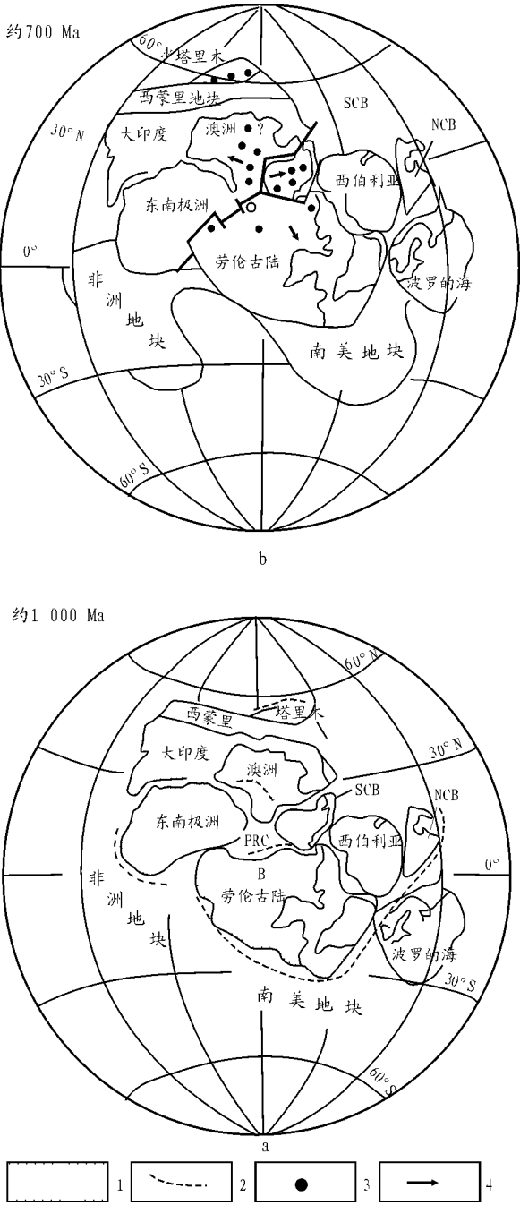
图 1 东亚克拉通 Rodinia 超大陆中的位置及变化 [15] 1. 格伦威尔期活动带;2. 格伦威尔期俯冲带;3. 冰川发生地; 4. 板块运动方向 NCB—华北地块;SCB—华南地块;PRC—普斯特河杂岩; B—贝尔特盆地 Fig. 1 Location and variation of East Asia Cratons in the Rodinia Super Continent
