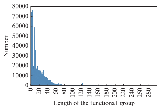
图 3 USPTO 数据集克级分子式官能团长度分布图
