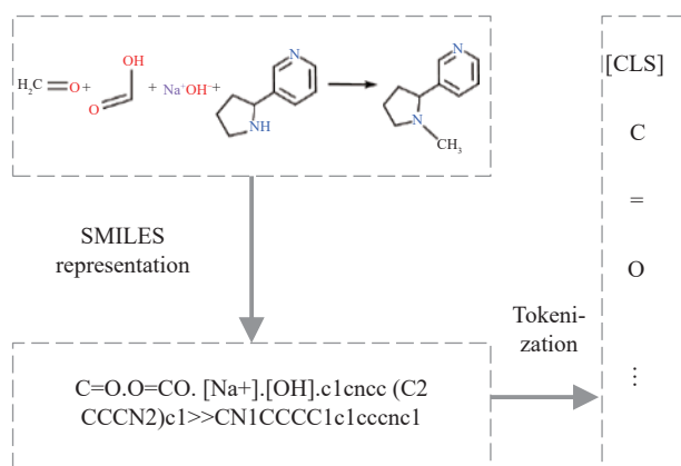
图 1 化学反应分子式的 SMILES 格式转化与分词示意图
