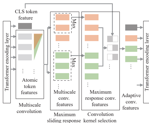
图 2 自适应卷积模块示意图
