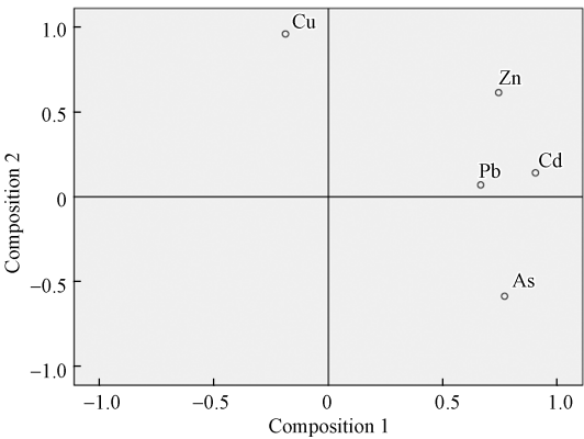
图 1 土壤 5 种重金属载荷散点图
