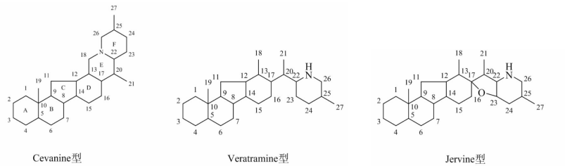
图 1 异甾体生物碱骨架结构
