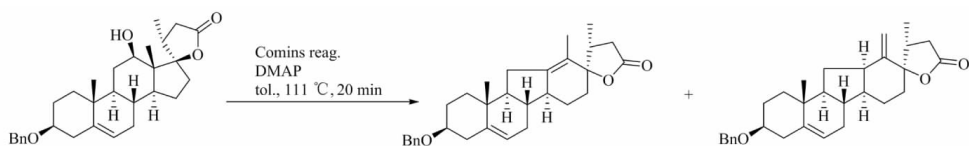
图 6 C-nor-D-homo-环合成
