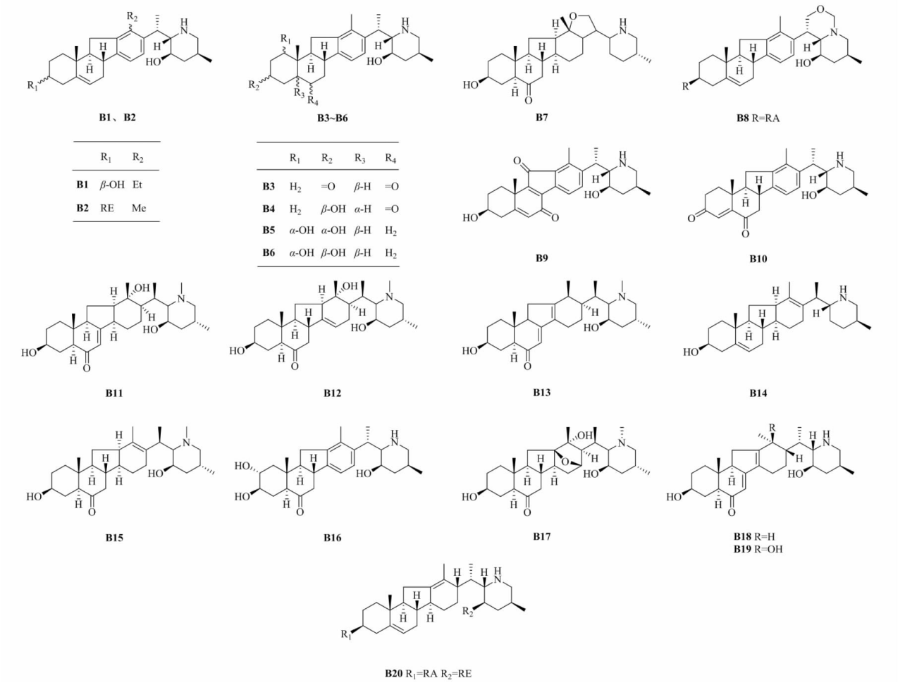
图 3 新发现 veratramine 型生物碱的化学结构
