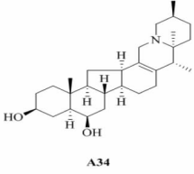
图 2 新发现 cevanine 型生物碱的化学结构
