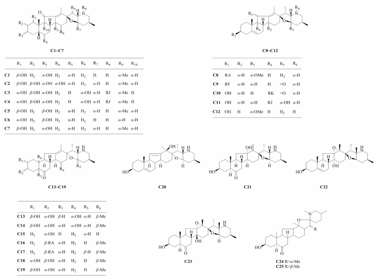
图 4 新发现 jervine 型生物碱的化学结构
