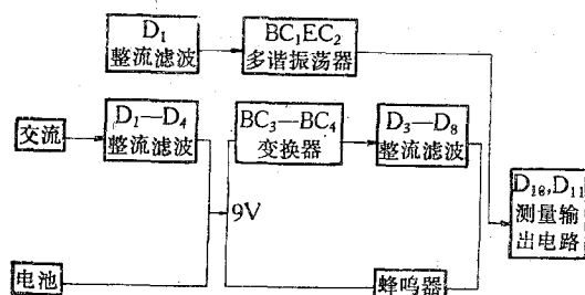
DL-3型698点送治疗机工作原理方框图
