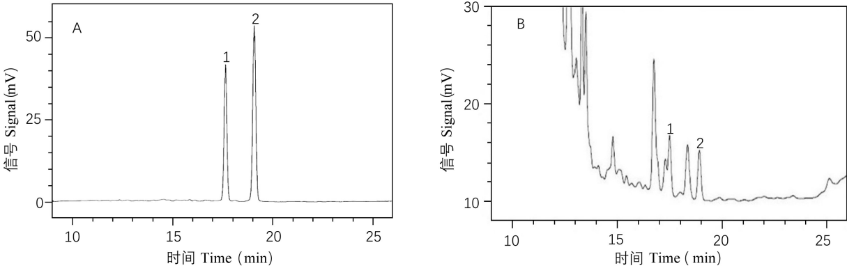
1. 柠檬苦素;2. 诺米林。 1. Limonin; 2. Nomilin.
