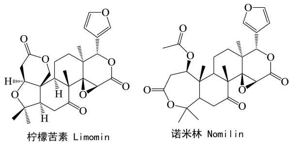
图 1 柠檬苦素和诺米林的化学结构式
