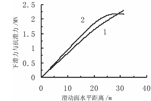
图 5 沿滑动面的抗滑力 R 和下滑力 T 的积分 1—抗滑力 R 的积分;2—下滑力 T 的积分
