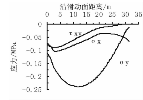
图 3 初始 C, \varphi 值时,沿滑动面的应力分布 \sigma_x, \sigma_y, \tau_{xy} 分别为正应力和剪应力
