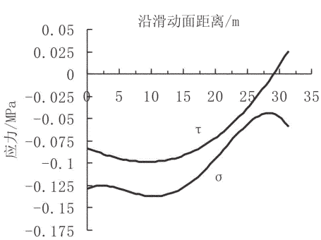
图 4 初始 C, \varphi 值时,垂直于滑动面的法向应力 \sigma 和平行于滑动面的剪应力 \tau
