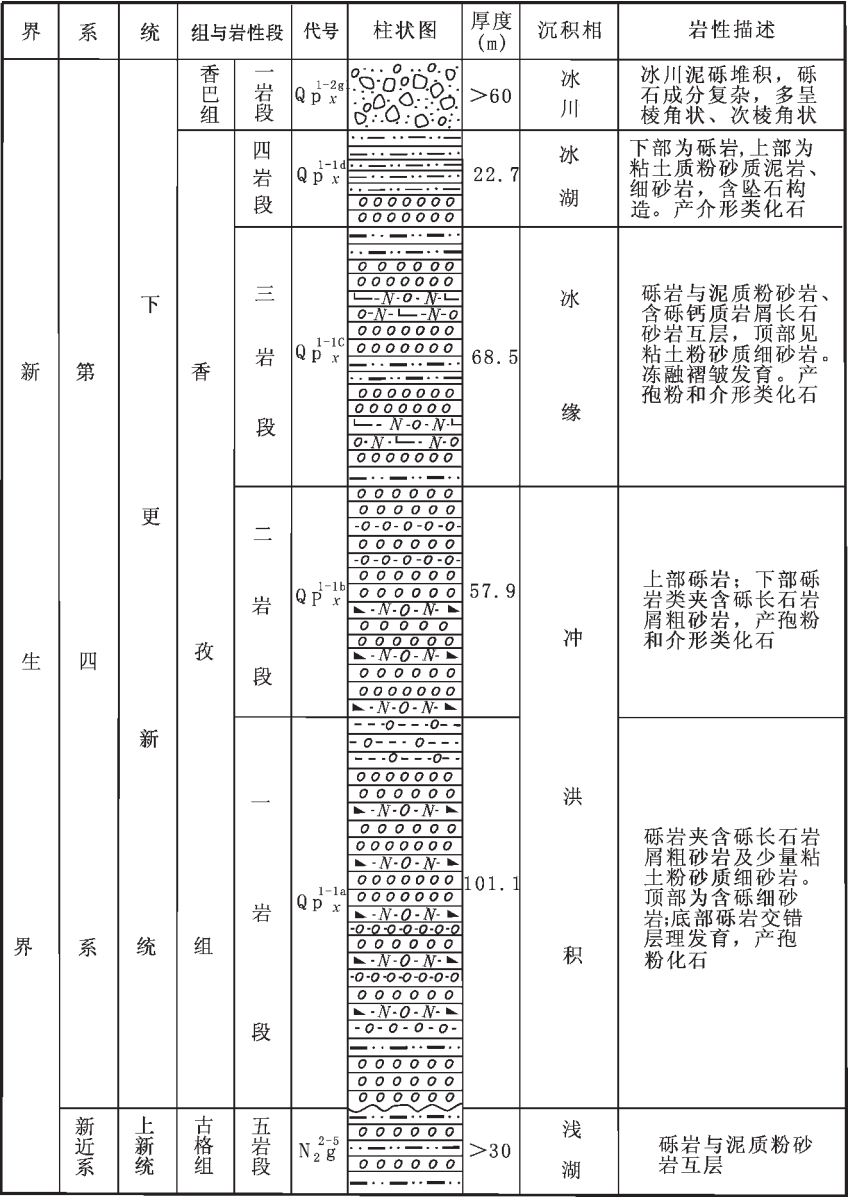
图 2 札达下更新统香孜组地层柱状图
