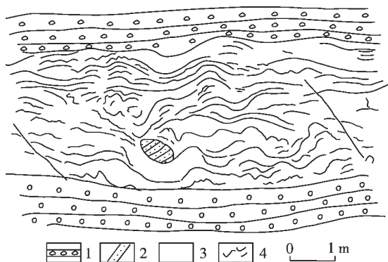
图 4 香孜组三岩段( Qp^{1-3x} )中发育的冻融褶皱
