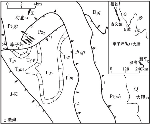
图1 漾濞县李子坪蛇绿混杂岩区域地质图
