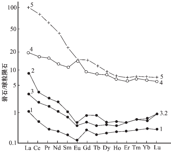
图3 李子坪蛇绿混杂岩稀土元素分布型式
