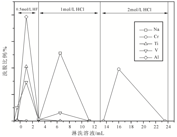
图 3 第二步化学分离淋洗曲线 Fig. 3 Elution curves of elements in column 2
