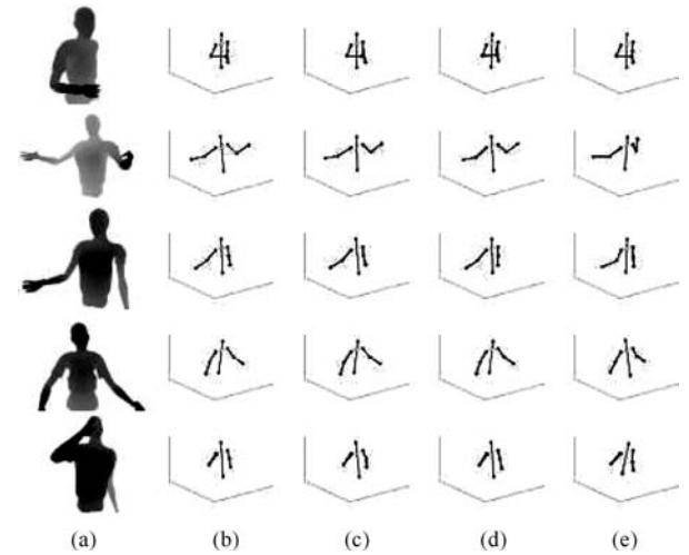
图 10 合成数据集上的姿态估计结果 ((a) 深度图像; (b) 误分类处理前的结果; (c) Kmeans 处理后的结果; (d) 多级随机森林整合后的结果; (e) groundtruth)
