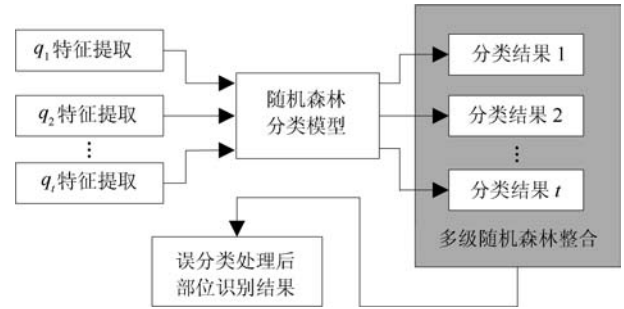
图 6 多级随机森林整合算法流程图
