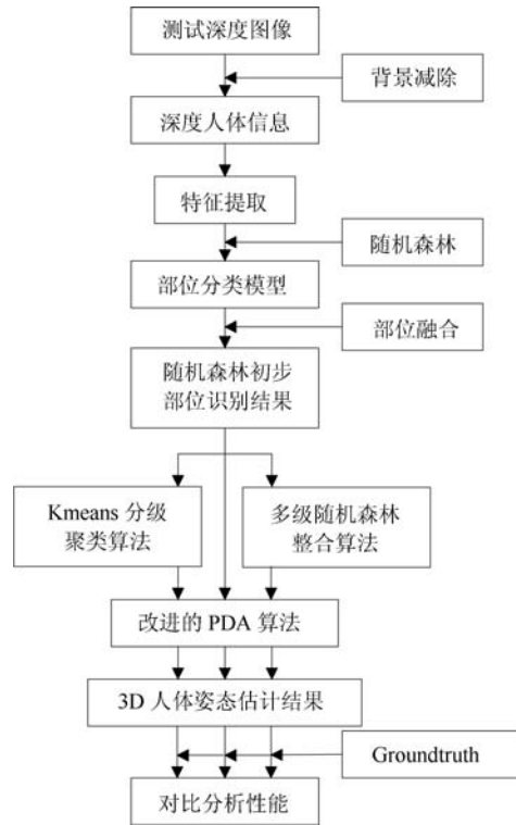
图 2 算法整体流程图
