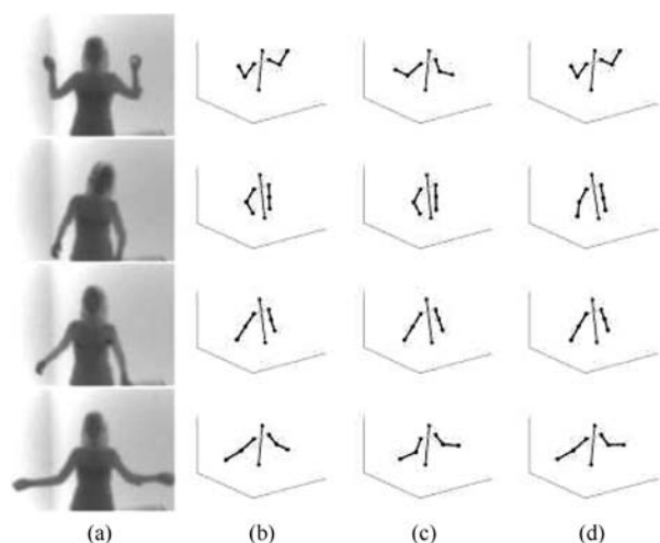
图 12 实际拍摄的深度图像上的姿态估计结果 ((a)~(d) 算法同图 10(a)~(d))
