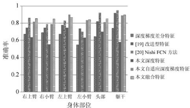
图 7 不同特征提取方法的部位分类结果对比
