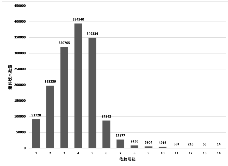
图 4 log4j-core 组件的层级依赖数量, 数据表明下游依赖组件多分布于前五层, 相对而言漏洞更易被触发
