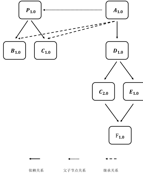
图 1 组件版本依赖关系示例图
