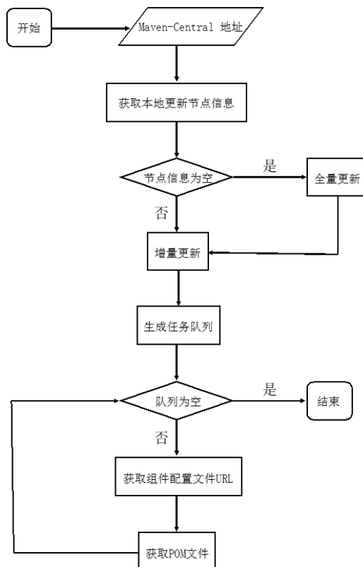
图3 Maven 组件配置信息爬虫工作流程图
