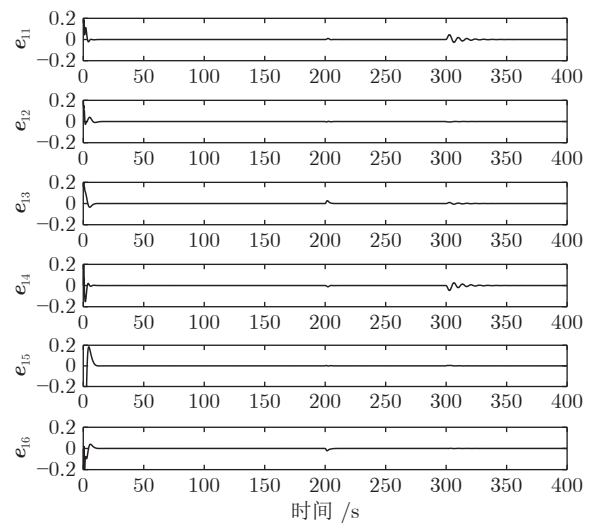
图 2 运动学状态误差 \mathbf{e}_1
