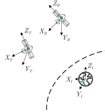
图 1 航天器近距离操作坐标系示意图
