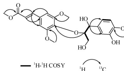
图 2 化合物 1 的 ^1\text{H} - ^1\text{H} COSY 相关和 HMBC 相关
