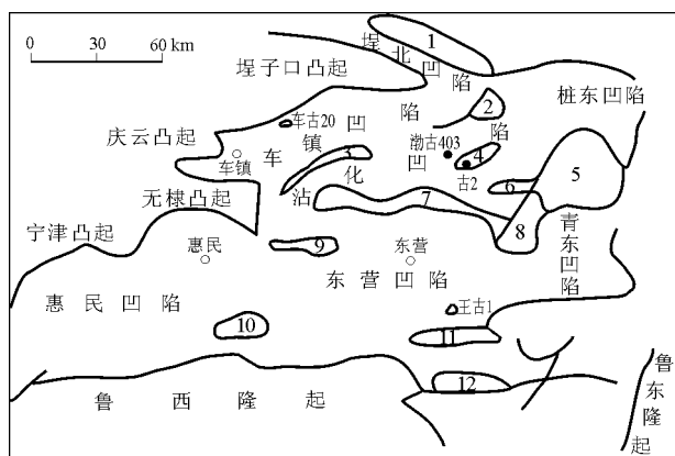
图1 渤海湾盆地济阳坳陷构造单元划分
