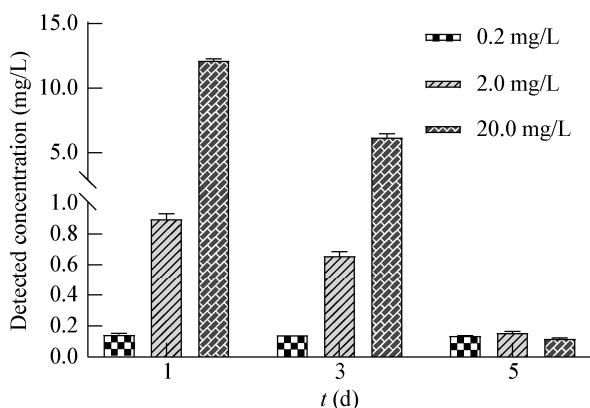
图 10 SPZ 实验组辛硫磷的降解
