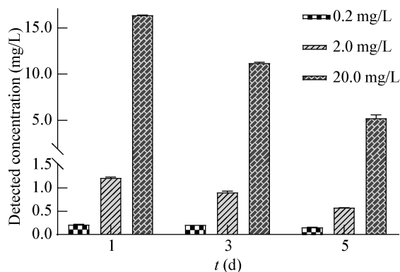
图 9 空白培养基中辛硫磷的降解
