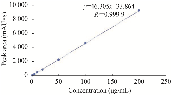
图 8 辛硫磷标准工作曲线 Figure 8 Standard curve of phoxim
