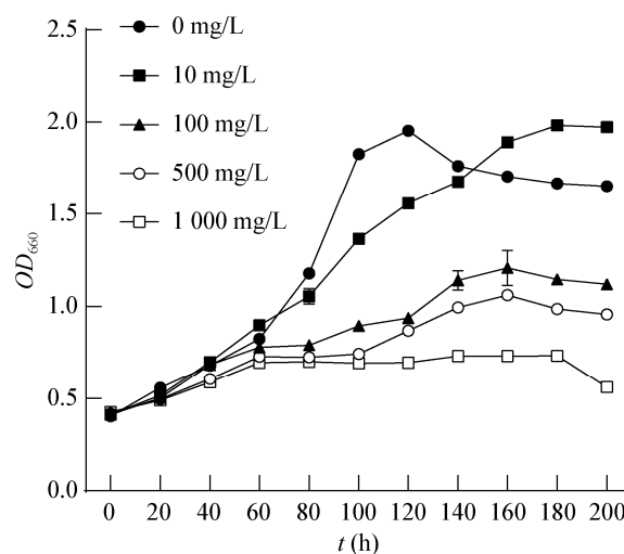
图 6 菌株 SPZ 在高浓度辛硫磷中的生长情况 Figure 6 Growth of strain SPZ in high concentration phoxim
