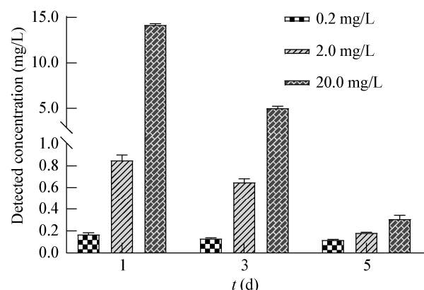
图 11 ST 实验组辛硫磷的降解
