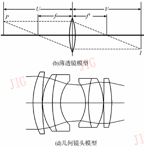
图 2 各种相机镜头模型的光学成像过程
