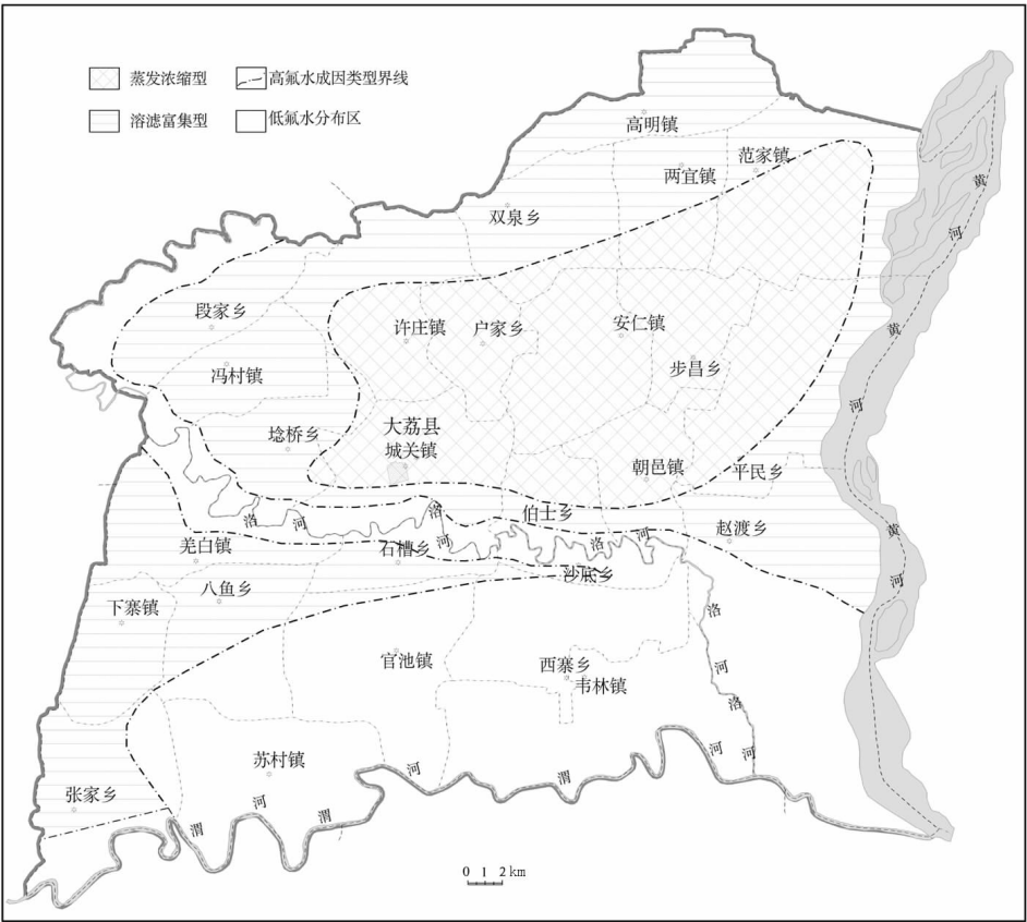
图 5 大荔县高氟地下水成因类型图 Fig.5 Genetic types of high-fluorine groundwater
