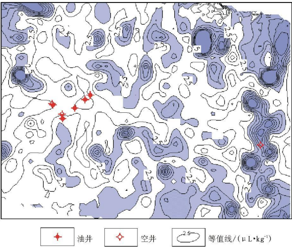
图 2 热释烃甲烷浓度等值线
