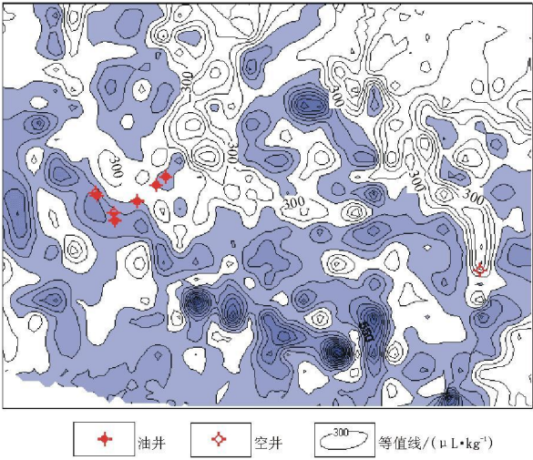
图 1 酸解烃甲烷浓度等值线
