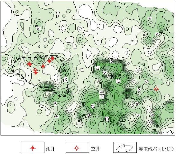
图 3 吸附烃甲烷浓度等值线
