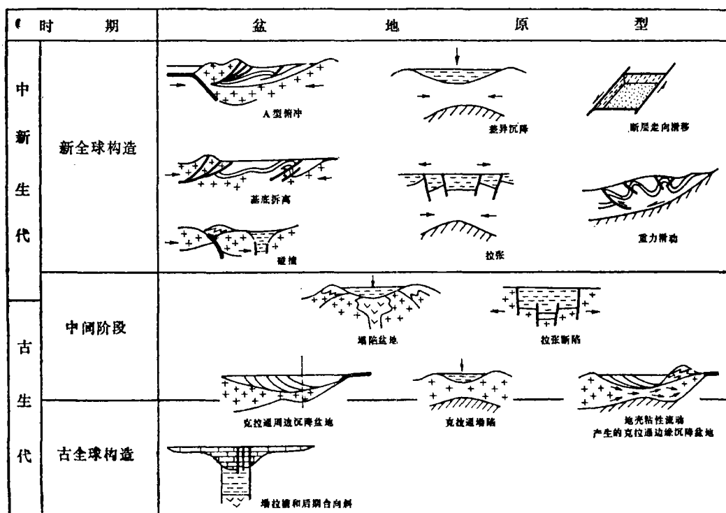
图1 不同时代的盆地原型示意图
