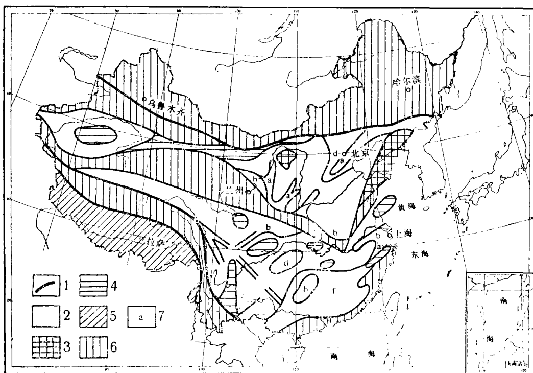
图2 中国古全球构造阶段和盆地分布图
