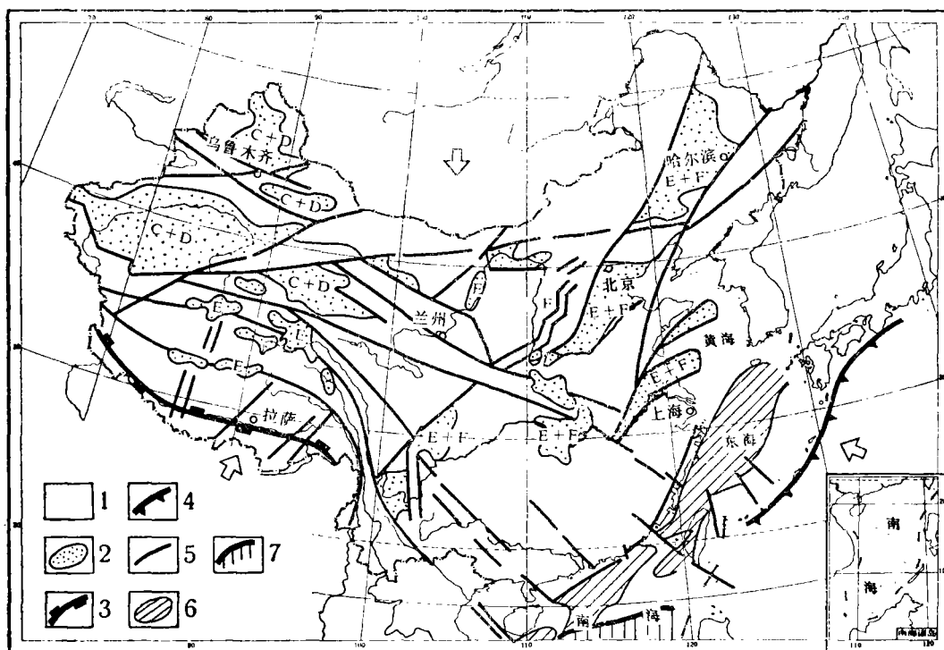
图5 中国新全球构造新生代阶段和盆地分布图
